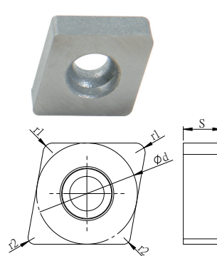
CNS1204
