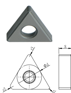
TNS1604
